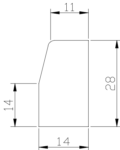
Bordillo 11x14x28x100
