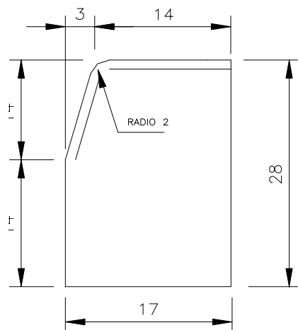
BORDILLO DE CALZADA C3
