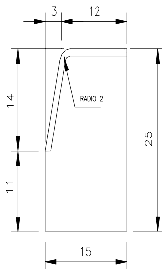
BORDILLO DE CALZADA C5
